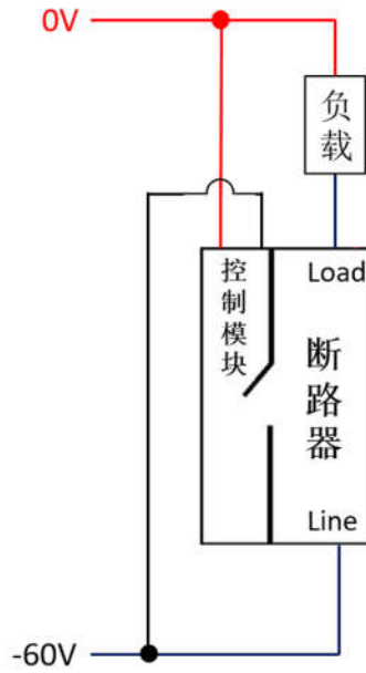
接线图
